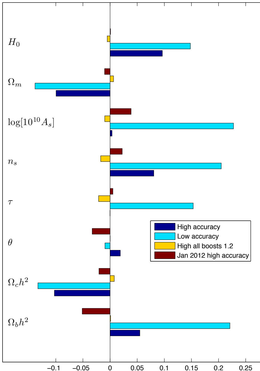
difference in posterior mean / error bar
